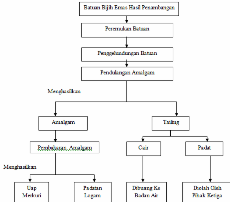
Gambar 5 Bagan Alir Proses Amalgamasi di Lokasi Penelitian
