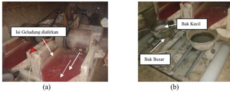
Gambar 3 Pendulangan Amalgam, (a) Amalgam dan Tailing Dituang Ke Bak (b) Bak Untuk Pendulangan Amalgam
