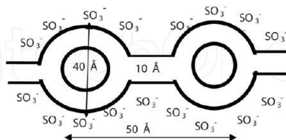
Fig. 4. Nafion cluster (Hamnett, 2003).
