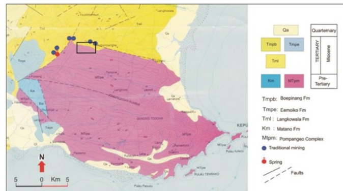
Gambar 2. Peta geologi daerah penelitian
