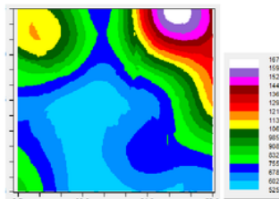
Gambar 4. Taksiran kriging penyebaran kadar emas plaser
