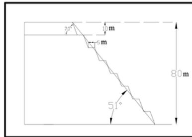
Gambar 3. Dimensi Jenjang Akhir Penambangan
