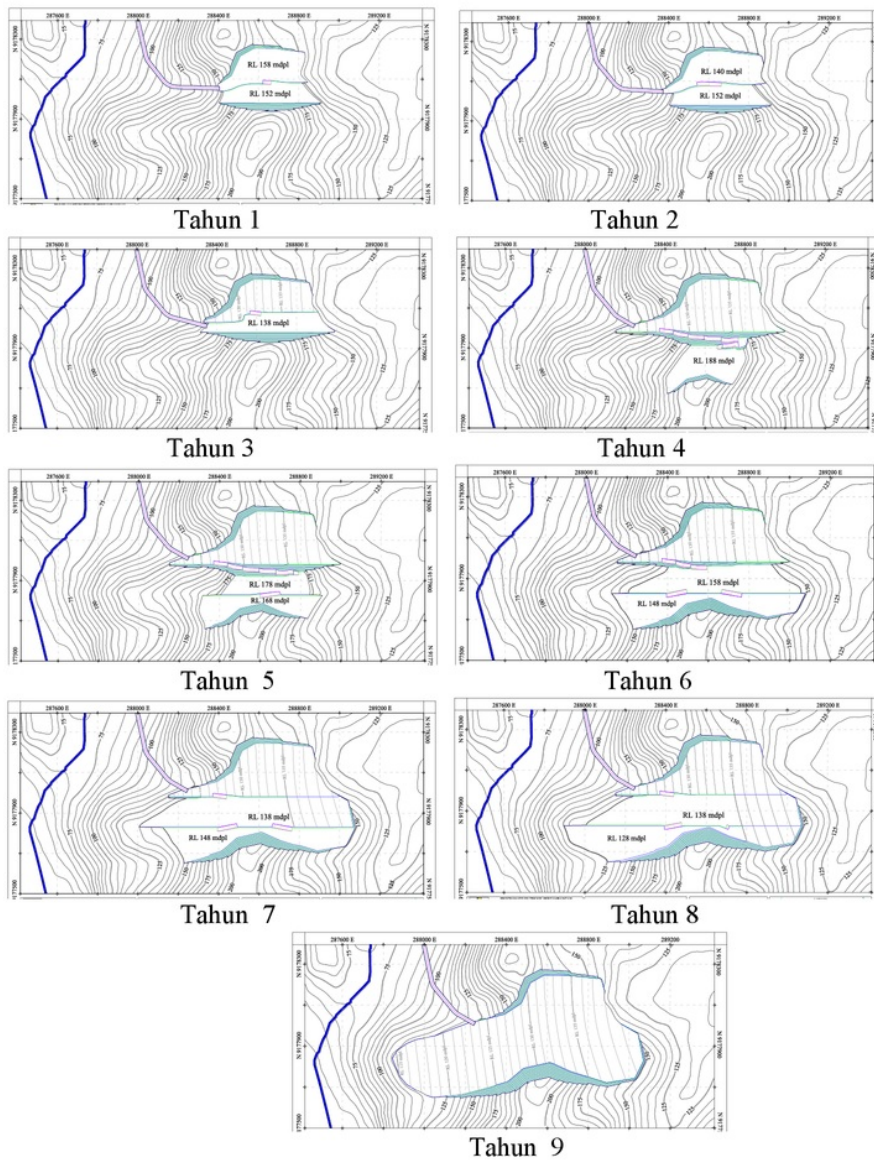
Gambar 4. Urut-urutan penambangan batugamping
