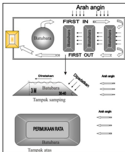
Gambar 12. Manajemen stockpile untuk menghindarkan fenomena spontaneous combustion
