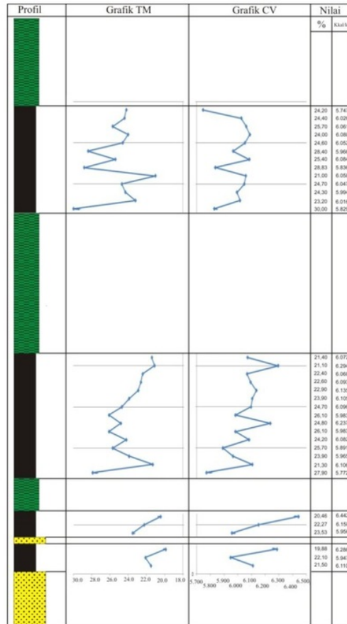
Gambar 9. Perkembangan CV-TM secara vertikal pada daerah penelitian
