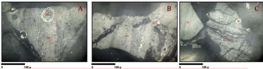
Gambar 3. (A) kenampakan reflektan semifusinite (Sf) dan telovitrinite (Te), (B) telovitrinite (Te), detrovitrinite (Dt) dan sclerinite (Sc), (C) sclerinitine (Sc) dan detrovitrinite (Te)
