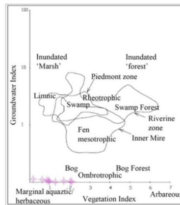
Gambar 6. Plotting lingkungan pengendapan pada diagram Calder
