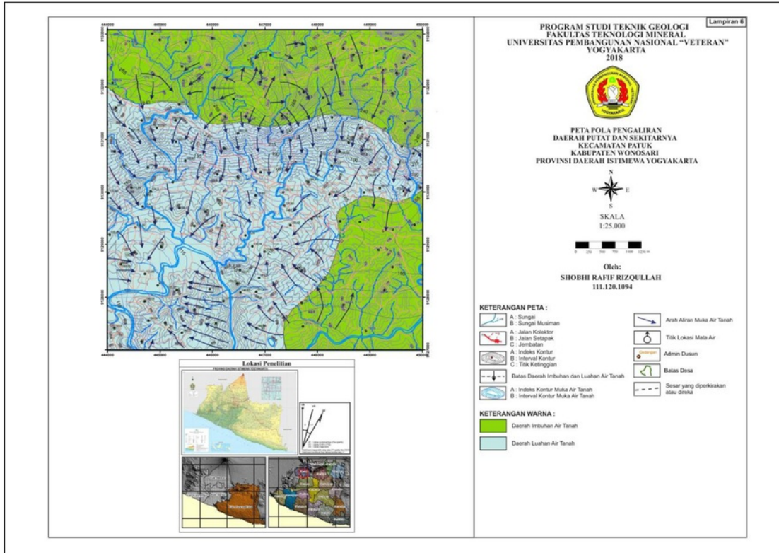
Gambar 6.a Peta Pola Pengaliran
