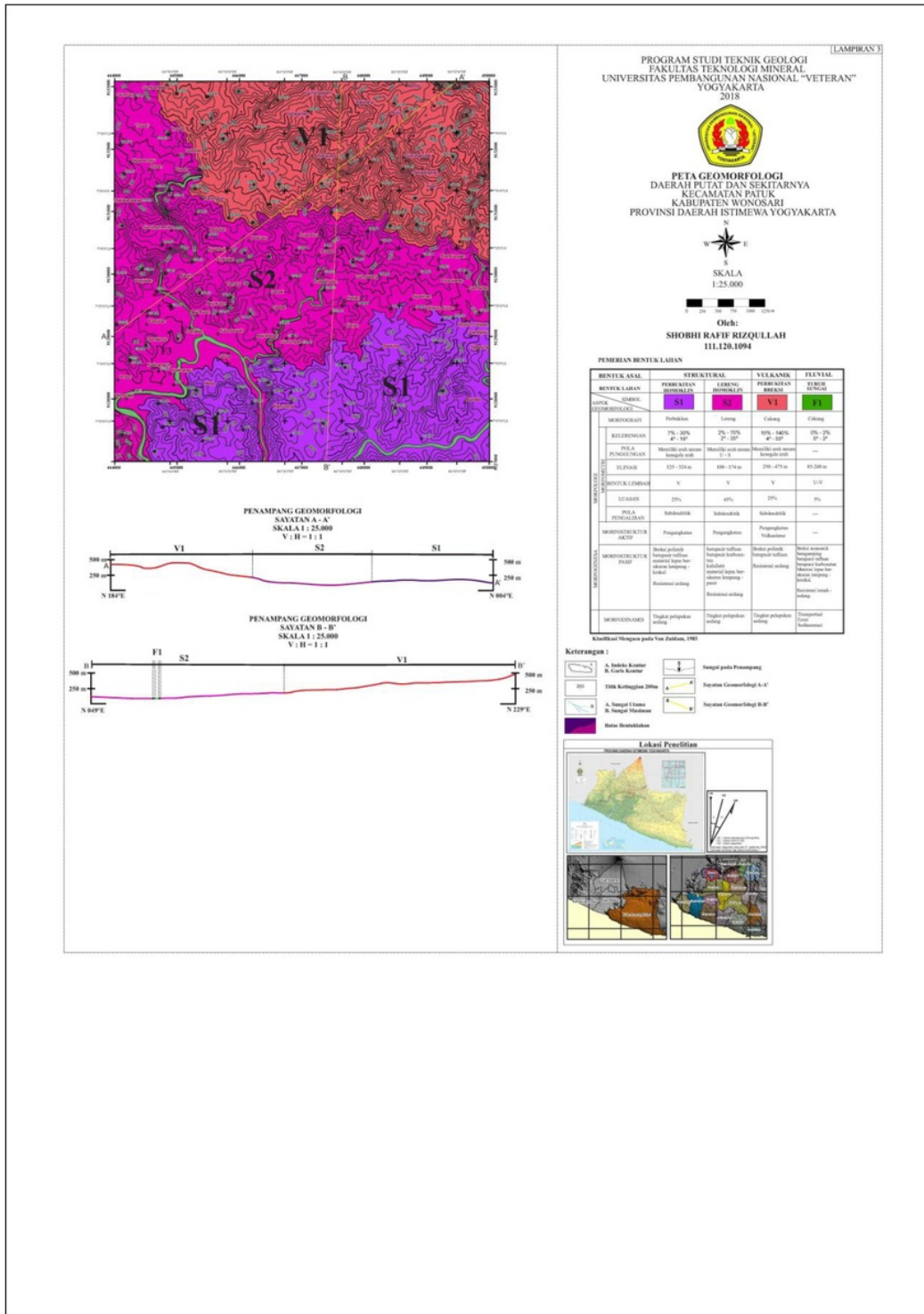
Gambar 7. Peta Geomorfologi
