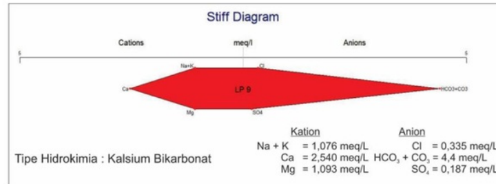
Gambar 1. Hasil analisis diagram stiff LP 9 daerah telitian.
