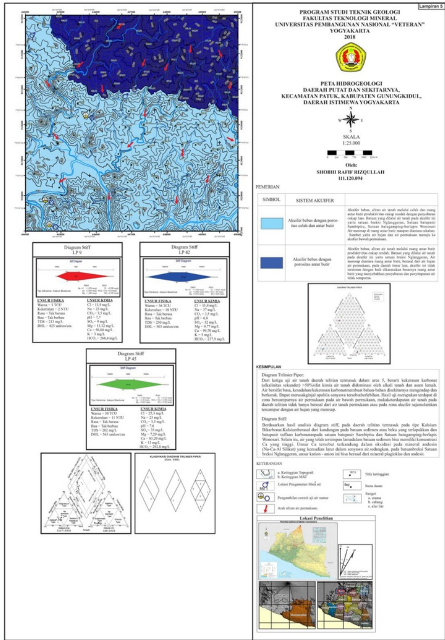
Gambar 9. Peta Hidrogeologi
