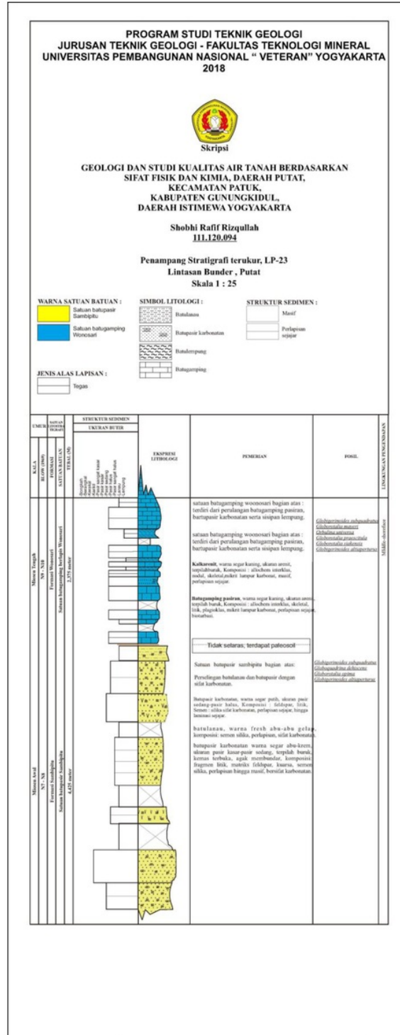
Gambar 10. Penampang Stratigrafi Terukur LP 23
