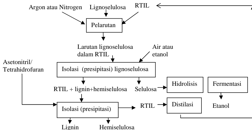
Gambar 3. Skema proses konversi lignoselulosa menjadi bioetanol.
