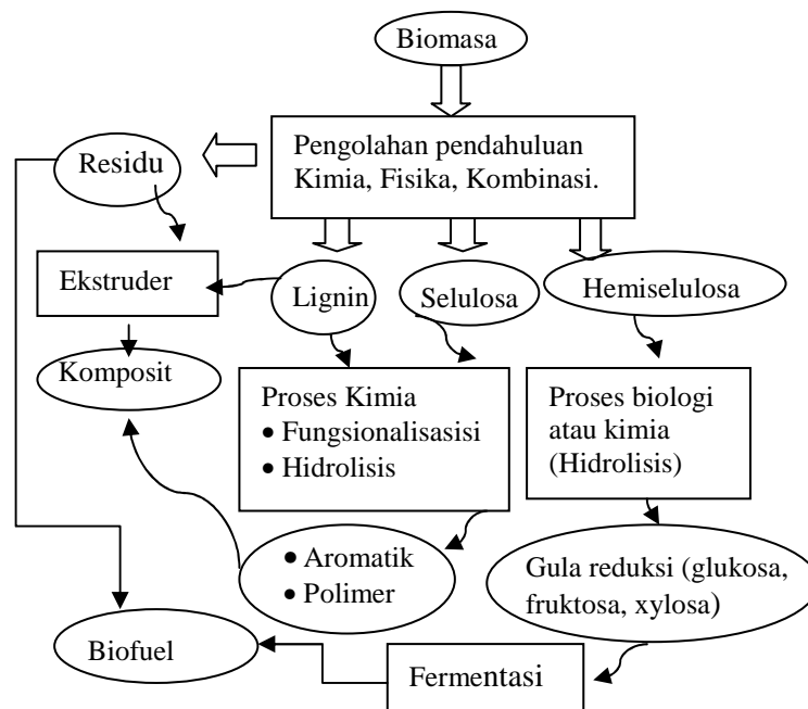
Gambar 1. Diagram alir konversi biomasa menjadi bahan bakar alkohol dan bahan kimia lain.
