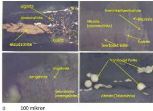
Gambar 4. Kenampakan mikroskopis batubara Seam Sangata
