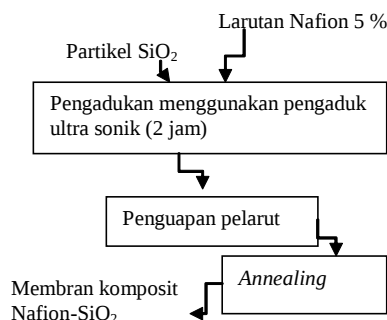
Gambar 2. Diagram alir sintesis membran komposit Nafion-SiO 2 metode dispersi
