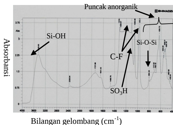
Gambar 6. Pola absorbansi terhadap bilangan gelombang hasil analisis FT-IR membran komposit Nafion-SiO 2 (TEOS/ Nafion =10/90 (berat/berat))
