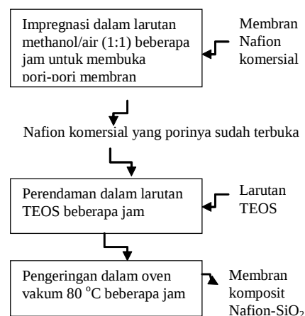
Gambar 1. Diagram alir sintesis membran komposit Nafion-SiO 2 metode impregnasi
