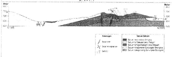
PENAMPANG GEOLOGI SAYATAN A-A' DAERAH PROSPEK RASIK SKALA 1 : 5.000 H. V. 1 : 1
