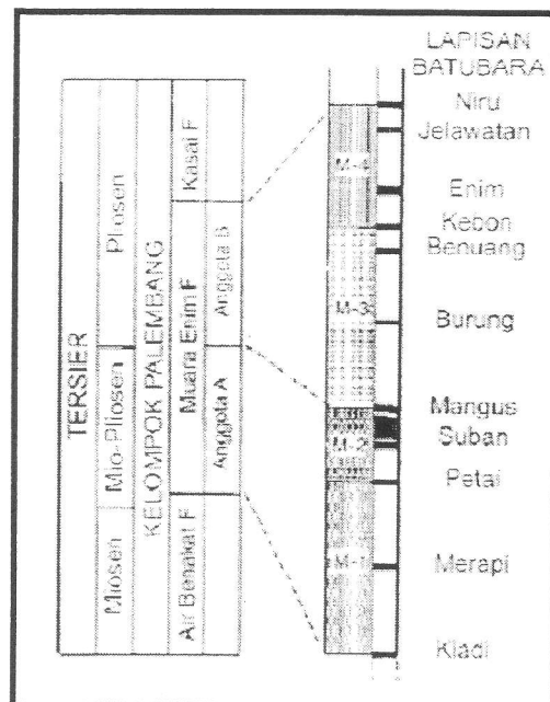
Gambar 3. Seam batubara anggota Formasi Muaraenim (Bamco, 1983)
