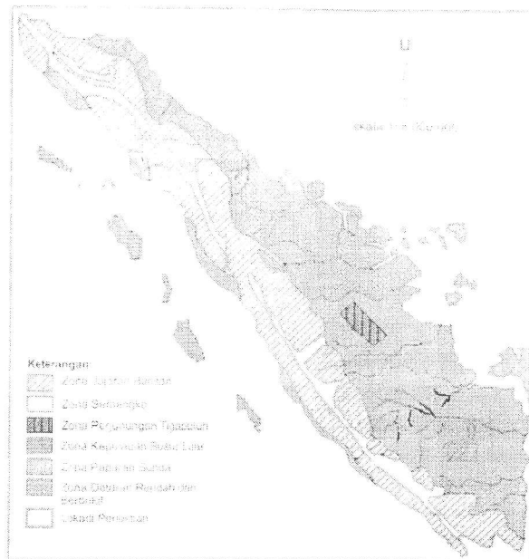
Gambar 2. Zona Fisiografi Pulau Sumatera (Bemmelen, 1949).
