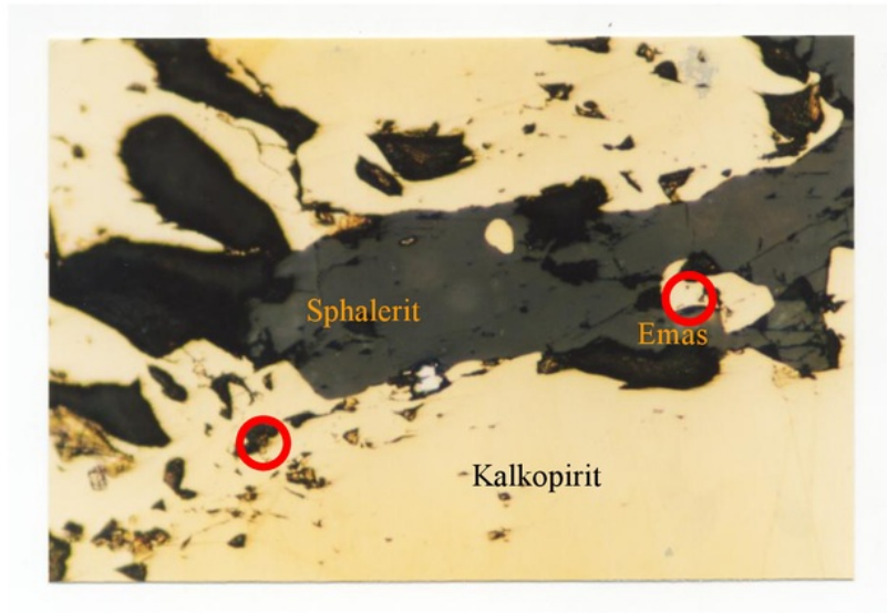
Foto 3. Sayatan mineragrafi Lokasi daerah Sangon terdapat mineral kalkopirit berwarna kuning dan sphalerit berwarna abu-abu biasanya hadir bersama emas elektrum .
