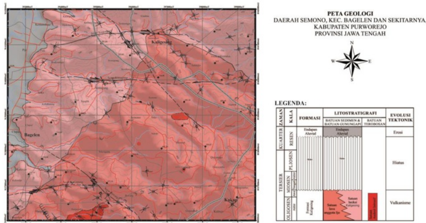
Gambar 6. Peta geologi daerah penelitian
