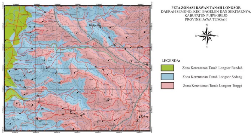
Gambar 9. Peta zonasi rawan longsor daerah penelitian
