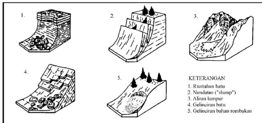
Gambar 4. Jenis-jenis gerakan massa (Hoek & Bray, 1981)
