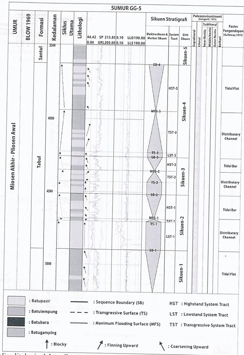
Gambar 5. Analisa litologi, elektrosikuen, system tract, unit sikuen dan lingkungan pengendapan sumur GG-5
