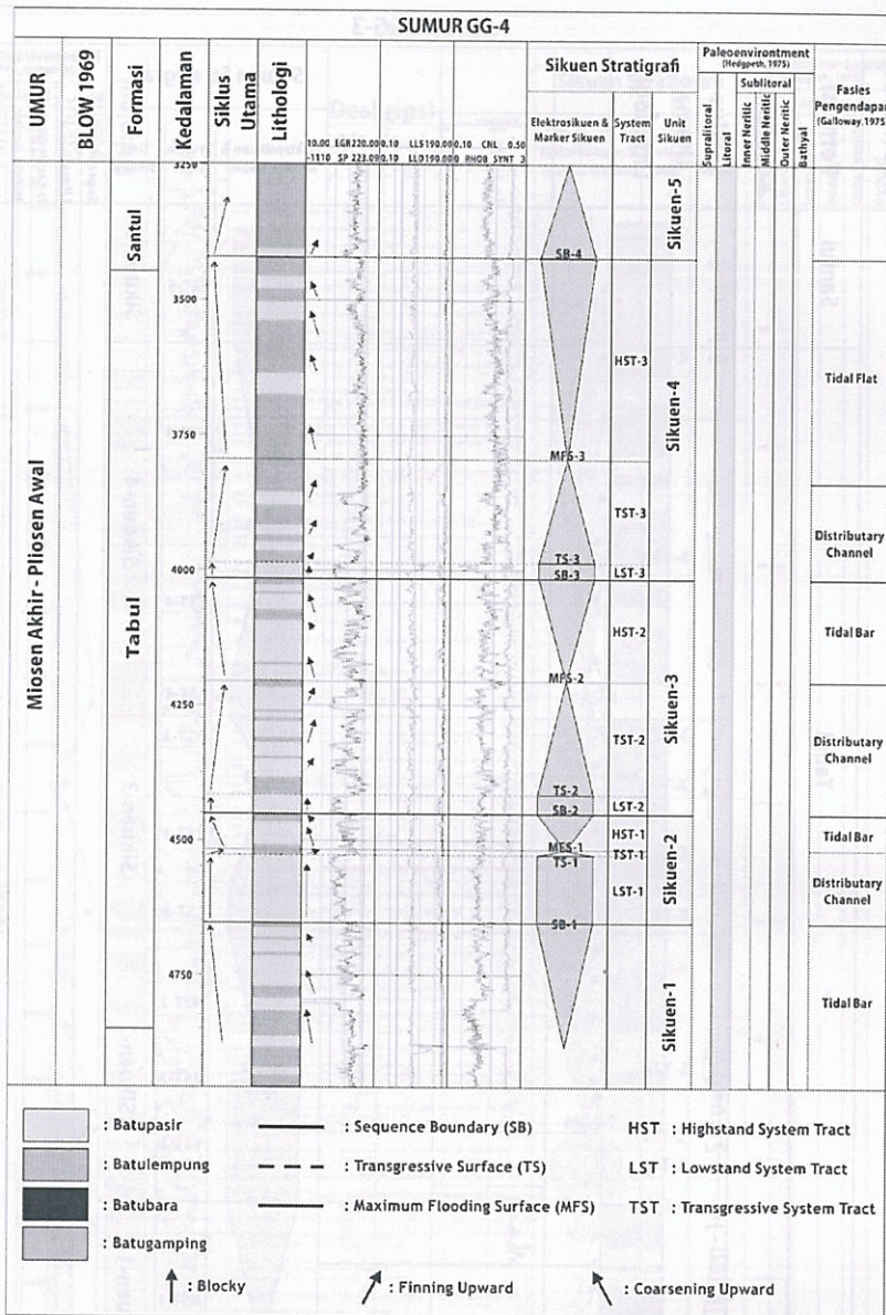
Gambar 4. Analisa litologi, elektrosikuen, system tract, unit sikuen dan lingkungan pengendapan sumur GG-4
