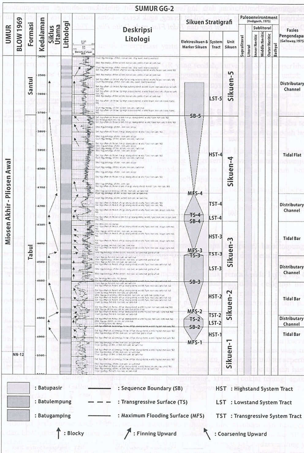
Gambar 2. Analisa litologi, elektrosikuen, system tract, unit sikuen dan lingkungan pengendapan sumur GG-2
