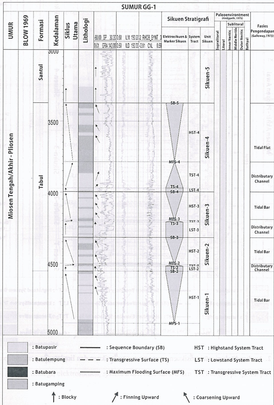
Gambar 1. Analisa litologi, elektrosikuen, system tract, unit sikuen dan lingkungan pengendapan sumur GG-1
