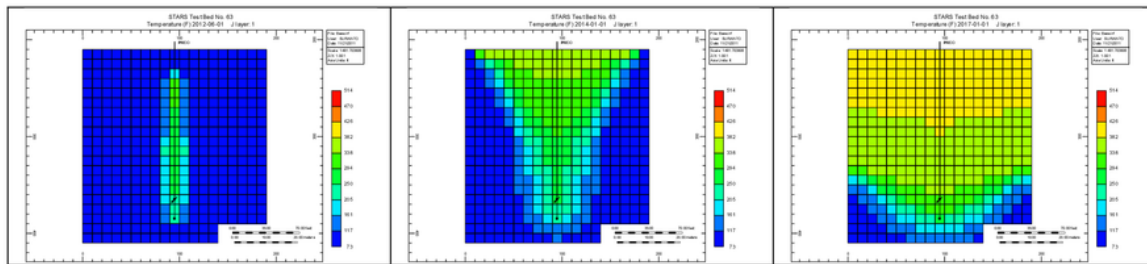
Gambar 7. Dsitribusi temperatur pada saat 6 bulan (a), 2 tahun (b) dan lima tahun (c) pada skenario base case
