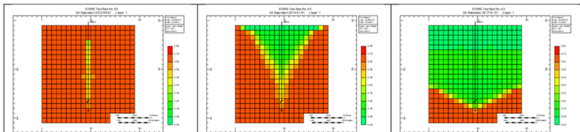
Gambar 8. Distribusi saturasi minyak pada saat 6 bulan (a), 2 tahun (b) dan lima tahun (c) pada skenario base case
