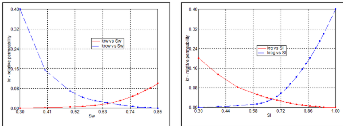
Gambar 5. Permeabilitas Minyak-air dan Minyak gas
