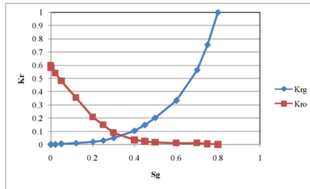
Gambar 8. Kurva Permeabilitas Relatif Gas-Minyak
