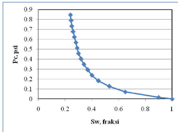
Gambar 9. Data Tekanan Kapiler Reservoir X
