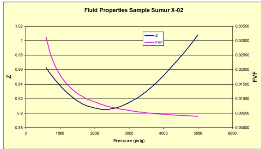
Gambar 6. Grafik korelasi factor Volume Formasi dan Z
