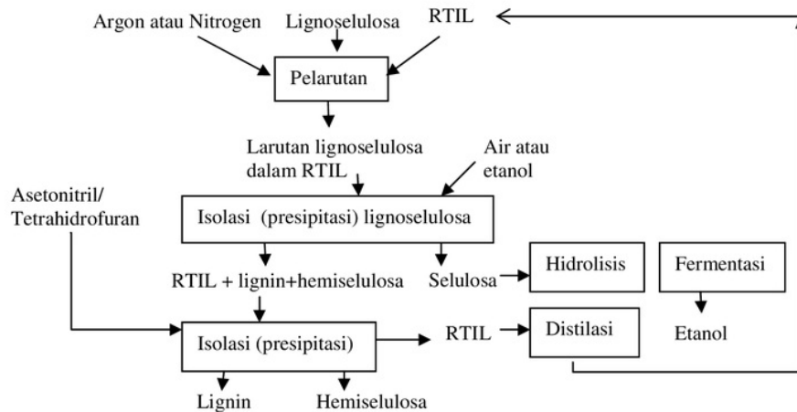
Gambar 3. Skema proses konversi lignoselulosa menjadi bioetanol.
