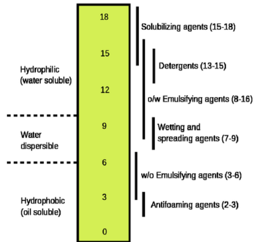
Gambar 2. Skala HLB dan Aplikasi Surfaktan
