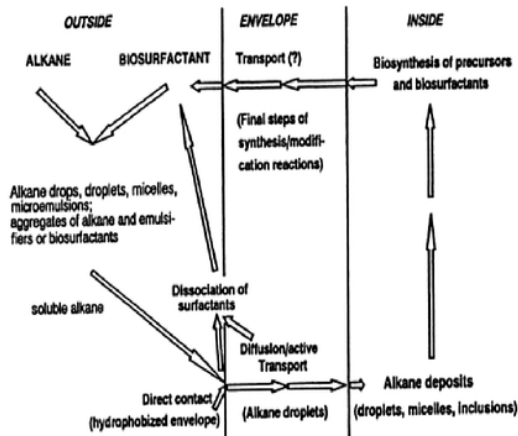
Gambar 6. Skema metabolisme sel dalam proses menghasilkan surfaktan.(Naim and Sukan, 1993).
