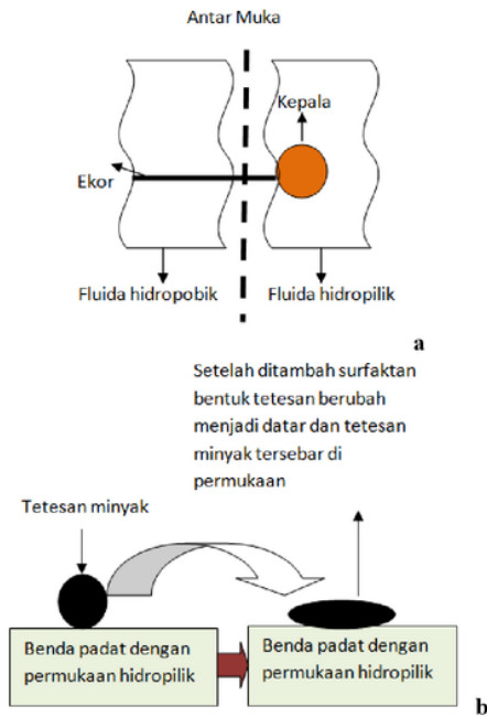
Gambar 1. Mekanisme Kerja Surfaktan
