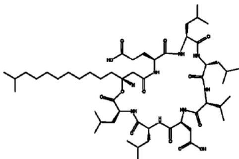
Gambar 3. Struktur kimia Surfactin (Lipopeptida) (Grau et al, 1999).
