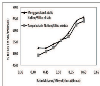
Gambar 4. Perbedaan % Berat biodisel dengan menggunakan katalis ganda dan katalis tunggal dengan perbandingan Metanol/minyak yang divariasi.
