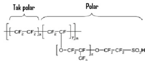
Gambar 1. Struktur Nafion.
