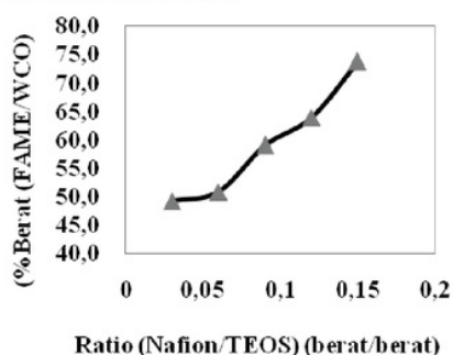
Gambar 3. Hubungan produk biodisel (% berat) dan konsentrasi Mafion dalam Nafion/TEOS.
