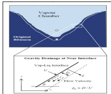
Gambar 2. Konsep dari Proses Gravity Drainage 2)
