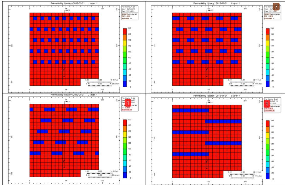
Gambar 9. Kondisi Barrier pada masing-masing skenario
