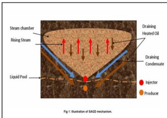
Gambar 3. Ilustrasi dari mekanisme SAGD 3)
