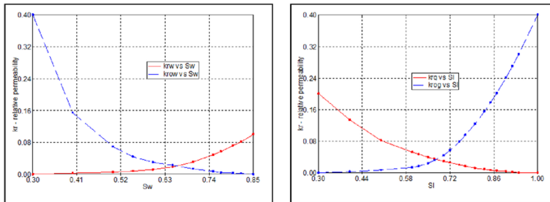
Gambar 5. Permeabilitas Minyak-air dan Minyak gas
