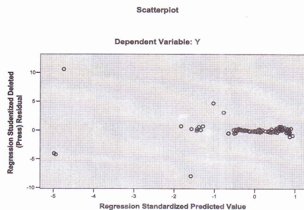
Gambar 3.2 Uji Heterokedastisitas
