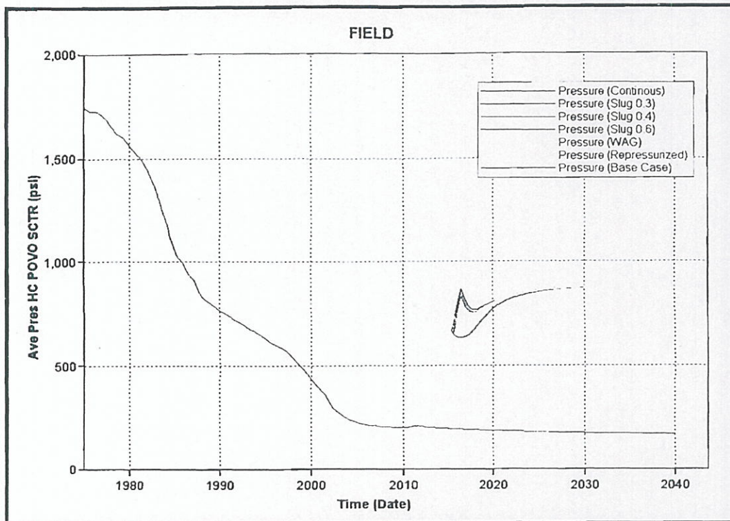
Gambar 6. Prediksi Tekanan Sumur Pilot EYK-176 pada Skenario Pilot
