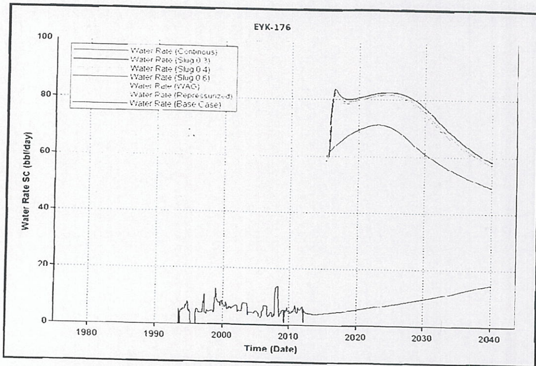
Gambar 4. Prediksi Laju Air Sumur Pilot EYK-176 pada Skenario Pilot
