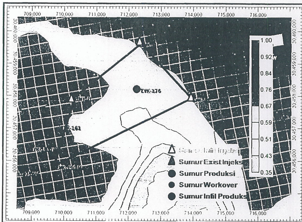
Gambar 1. Pola dan Lokasi Sumur Lapisan Y Lapangan X
