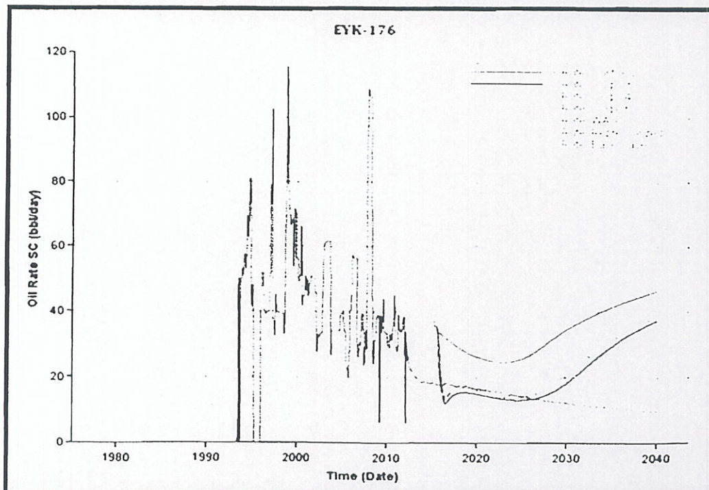
Gambar 3. Prediksi Laju Minyak Sumur Pilot EYK-176 pada Skenario Pilot
