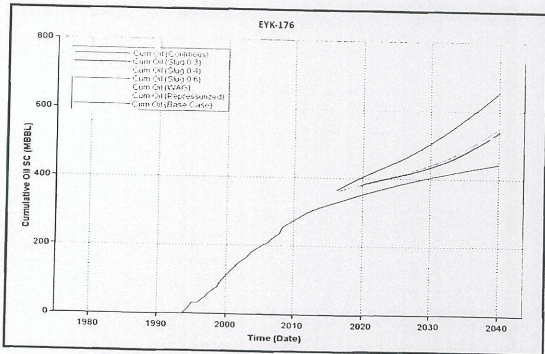
Gambar 5. Prediksi Komulatif Minyak Sumur Pilot EYK-176 pada Skenario Pilot
