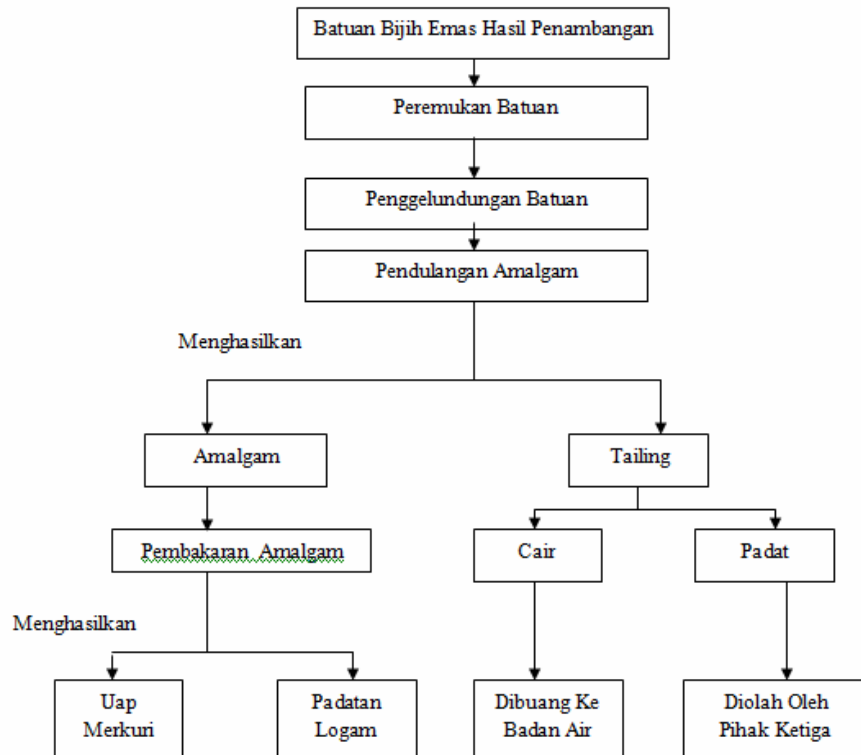
Gambar 5 Bagan Alir Proses Amalgamasi di Lokasi Penelitian
