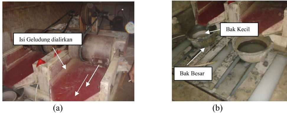
Gambar 3 Pendulangan Amalgam; (a) Amalgam dan Tailing Dituang Ke Bak (b) Bak Untuk Pendulangan Amalgam
