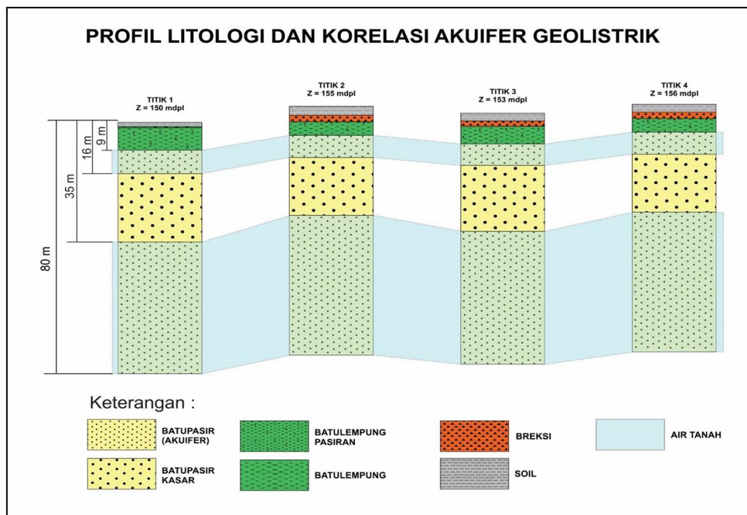
Gambar 4. Ilustrasi Penampang Korelasi Akuifer
