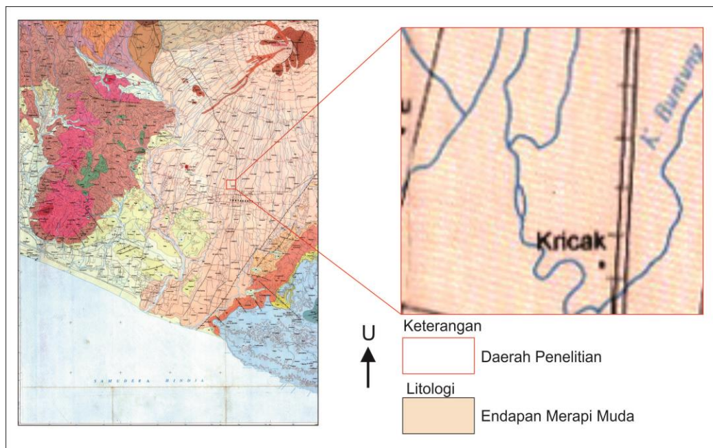
Gambar 1. Peta Geologi Daerah Telitian
