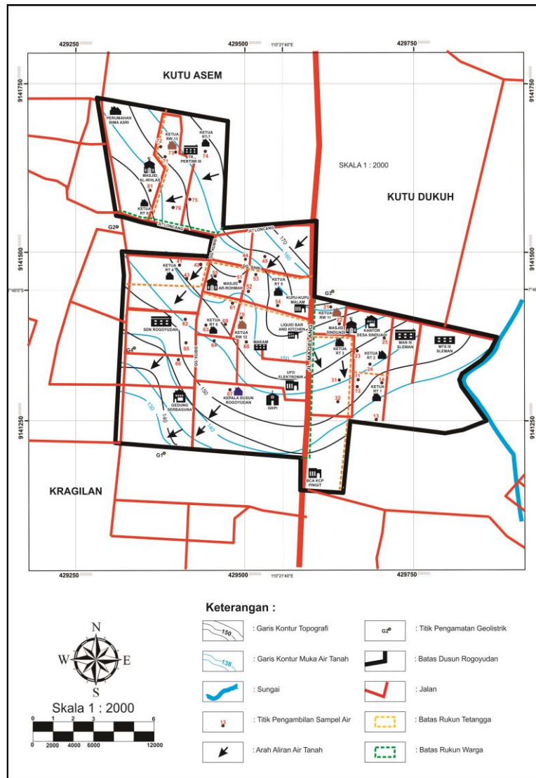
Gambar 5. Peta Muka Air Tanah dan Topografi di Dusun Rogoyudan
