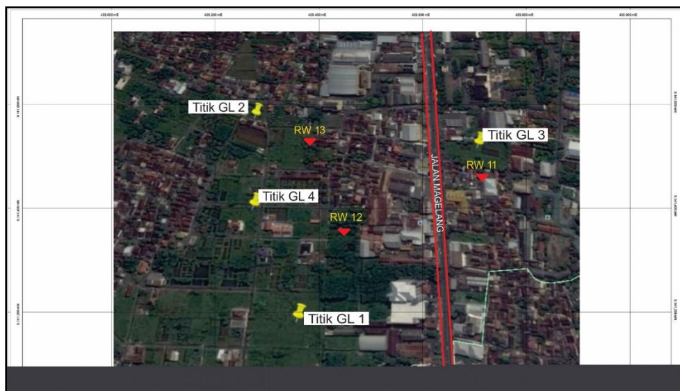
Gambar 2. Skema Penentuan Lokasi Titik Geolistrik
