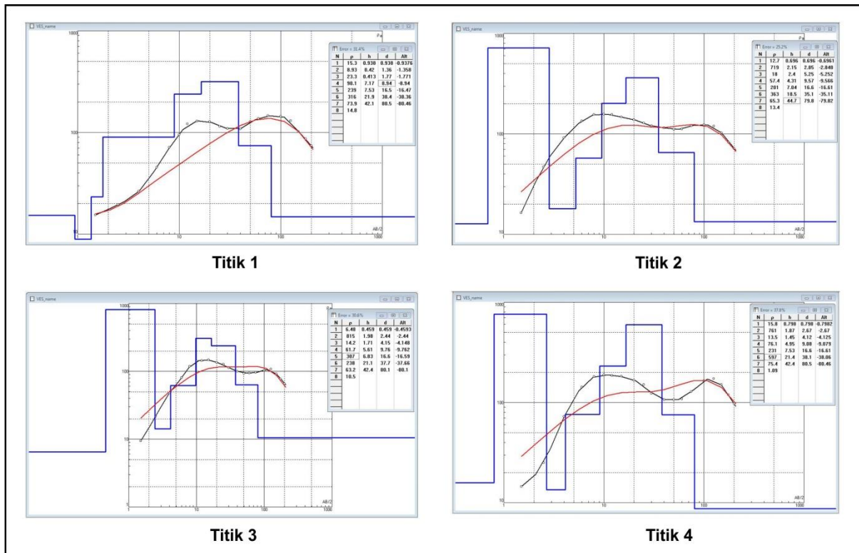
Gambar 3. Grafik IP2WIN pada 4 Titik Pengukuran Geolistrik metode Schlumberger
