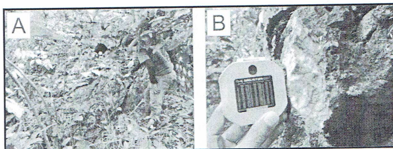
Gambar 3. (A) Singkapan Batugamping Sepingtang Berwarna Putih, Arah Kamera N 190° E ; (B) Close Up Singkapan, Arah Kamera N 182° E.
