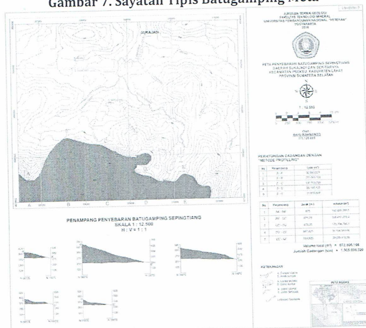
Gambar 8. Peta Sebaran dan Estimasi Cadangan Batugamping Sepingtiang
