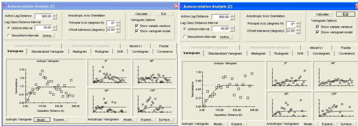
Gambar 4. Hasil variografi ketebalan batubara seam-A dan seam-B
