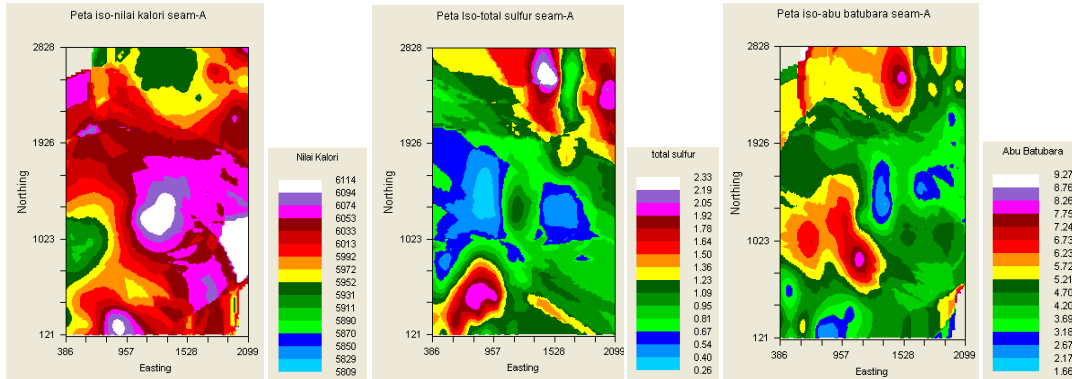
Lampiran 3. Hasil penaksiran nilai kalori, total sulphur, dan abu batubara seam-A memakai block kriging
