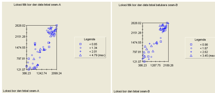
Gambar 1. Lokasi pemboran dan distribusi ketebalan batubara seam-A dan seam-B
