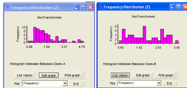
Gambar 2. Histogram ketebalan lapisan batubara seam-A dan seam-B
