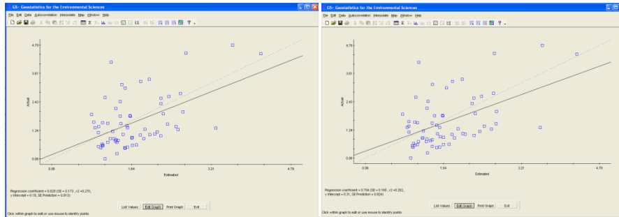
Gambar 8. Cross validation hasil penaksiran block dan point untuk batubara seam-A
