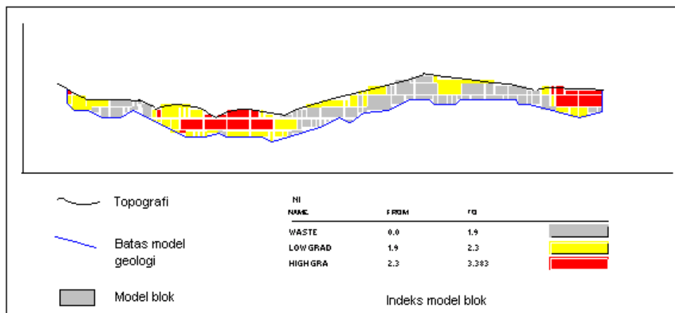
Gambar 7. Presentasi model pada penampang potong dengan koordinat N 4721° E
